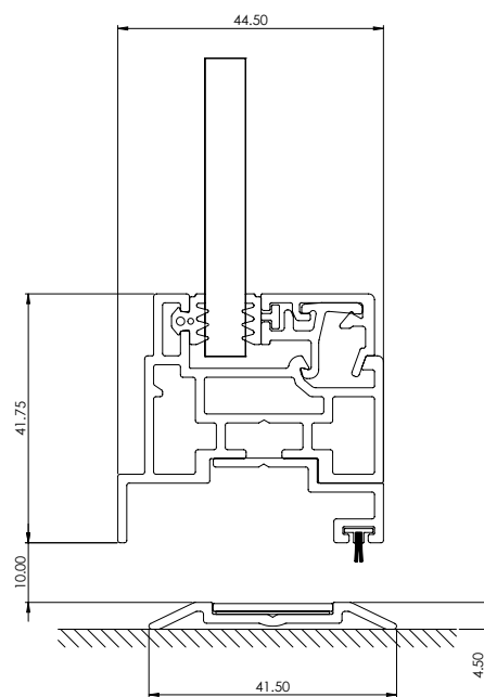
A-08854 DOOR BOTTOM SASH
