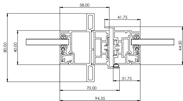
A-08850 SIDE LIGHT - DOOR
