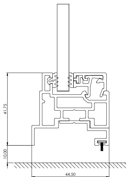
A-08853 DOOR BOTTOM SASH
