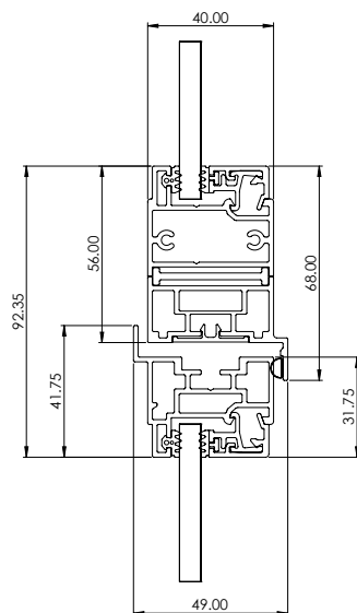
A-08849 TOP LIGHT - DOOR
